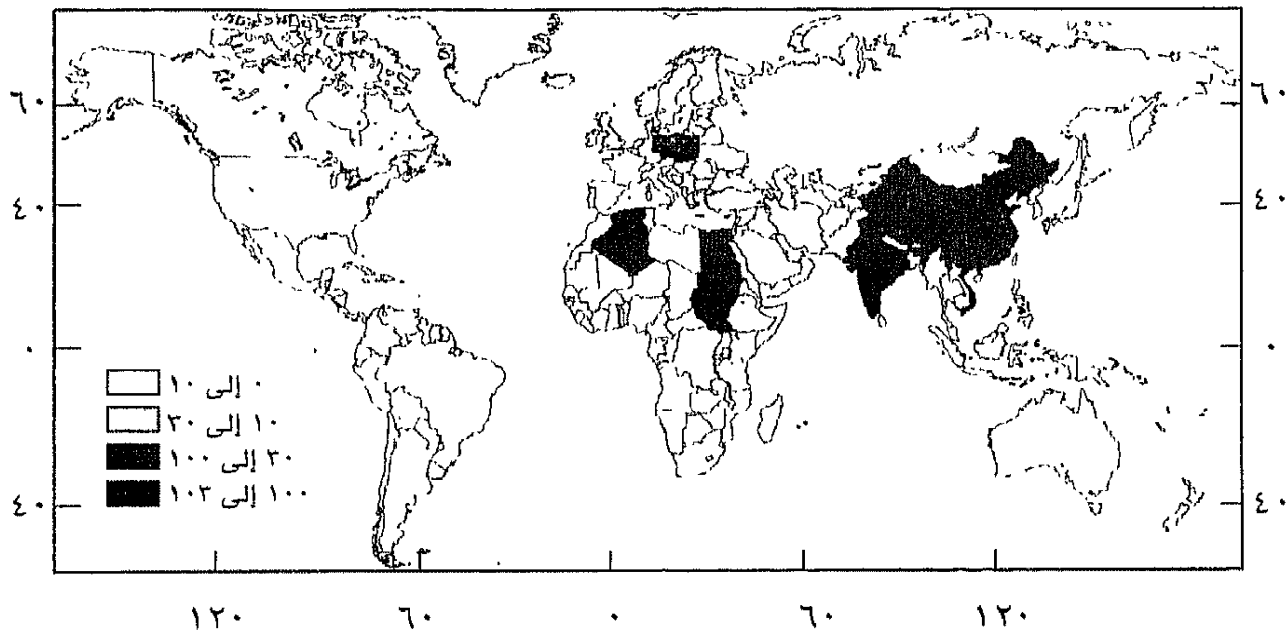
الشكل (٩.٢): جغرافيا الوجود العسكري السوفييتي مقاسا بمعدل الكثافة السنوي، ١٩٦٣ - ١٩٦٨ (من: Nijman 1992 b).
